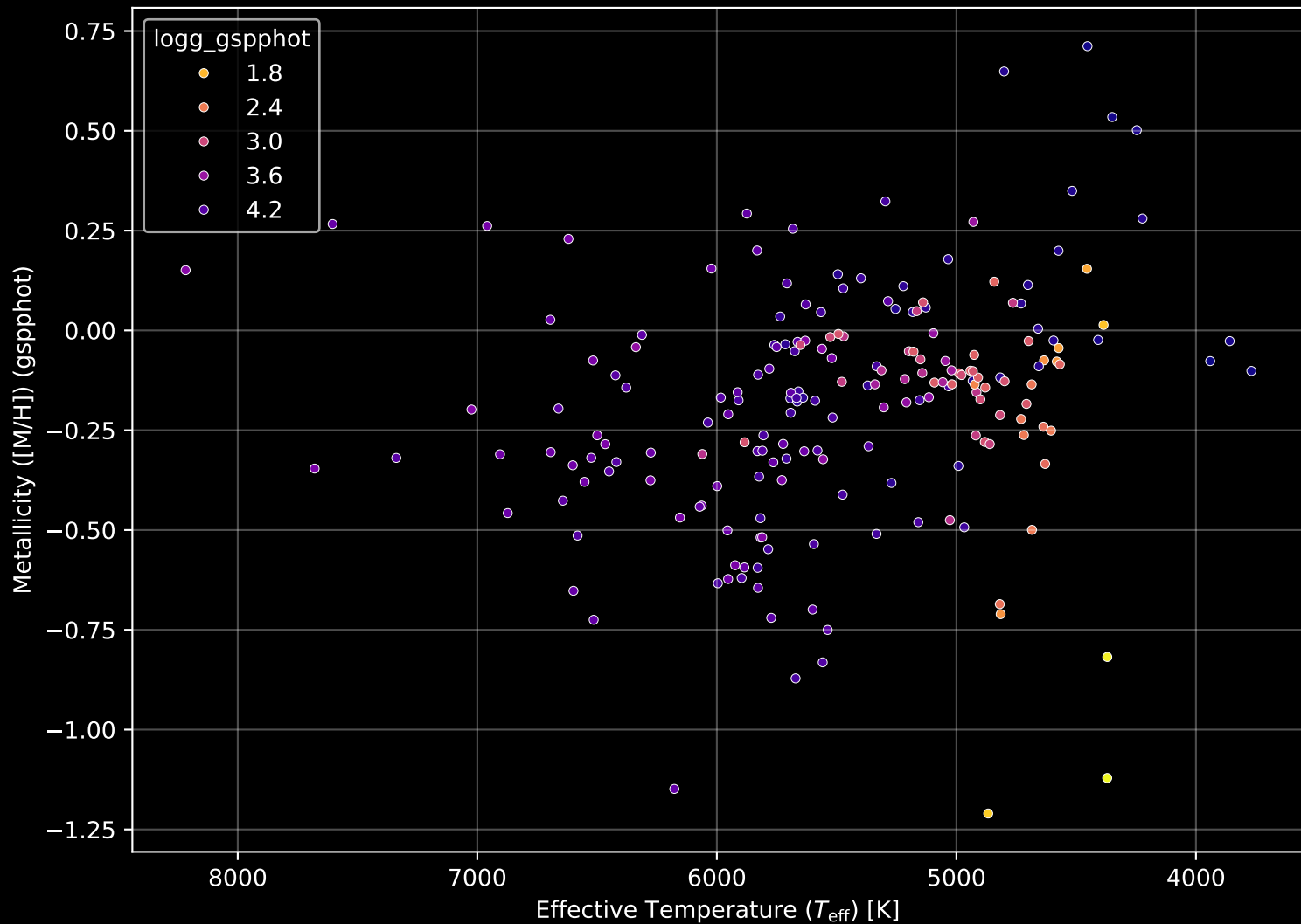
APOGEE DR17 Field: [075-35_MGA] Stellar Population Parameters (n= 199)
